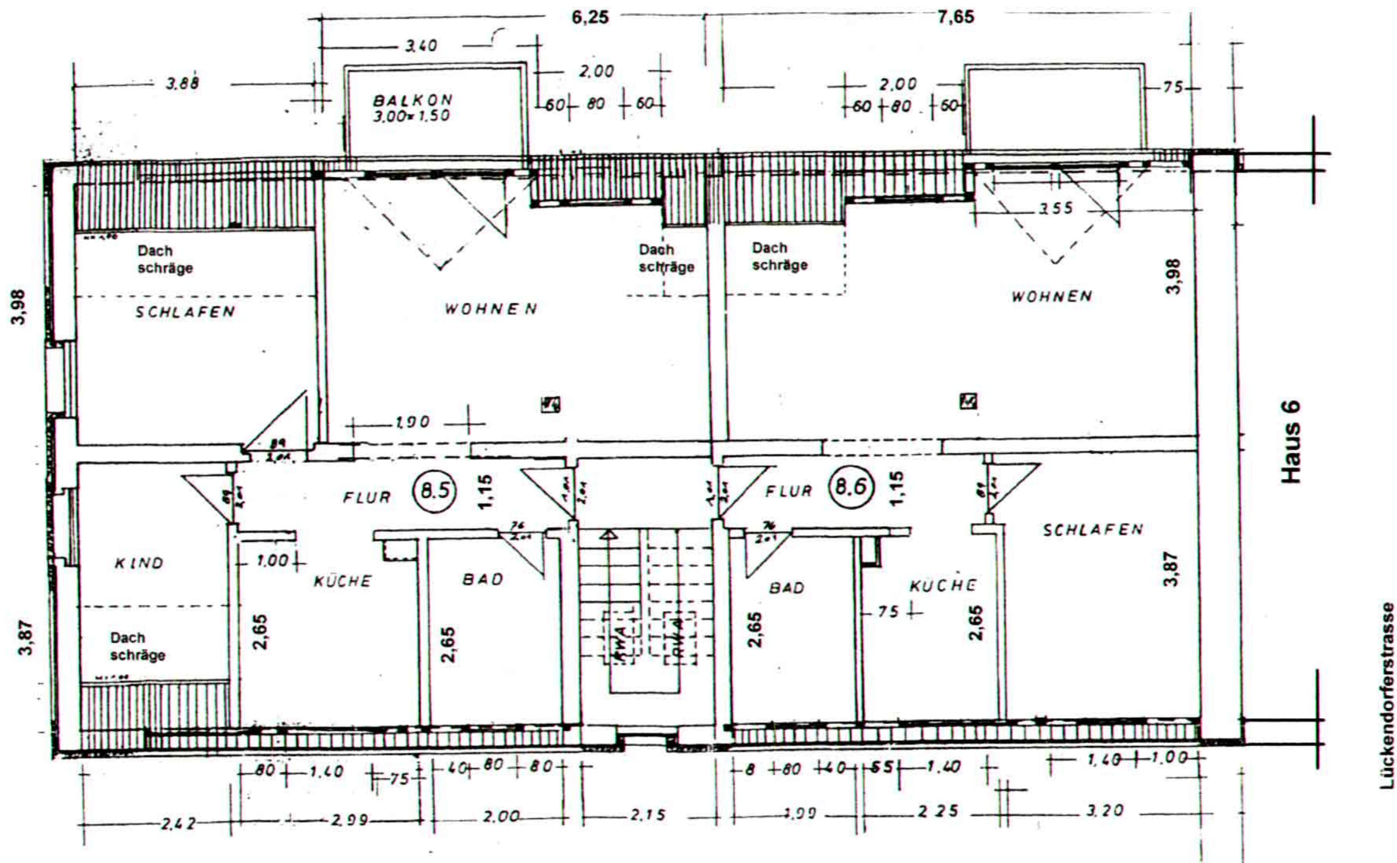
Oybin, Lückendorferstrasse 8 Grundriss Wohnungen 8.5 und 8.6 DACHGESCHOSS
