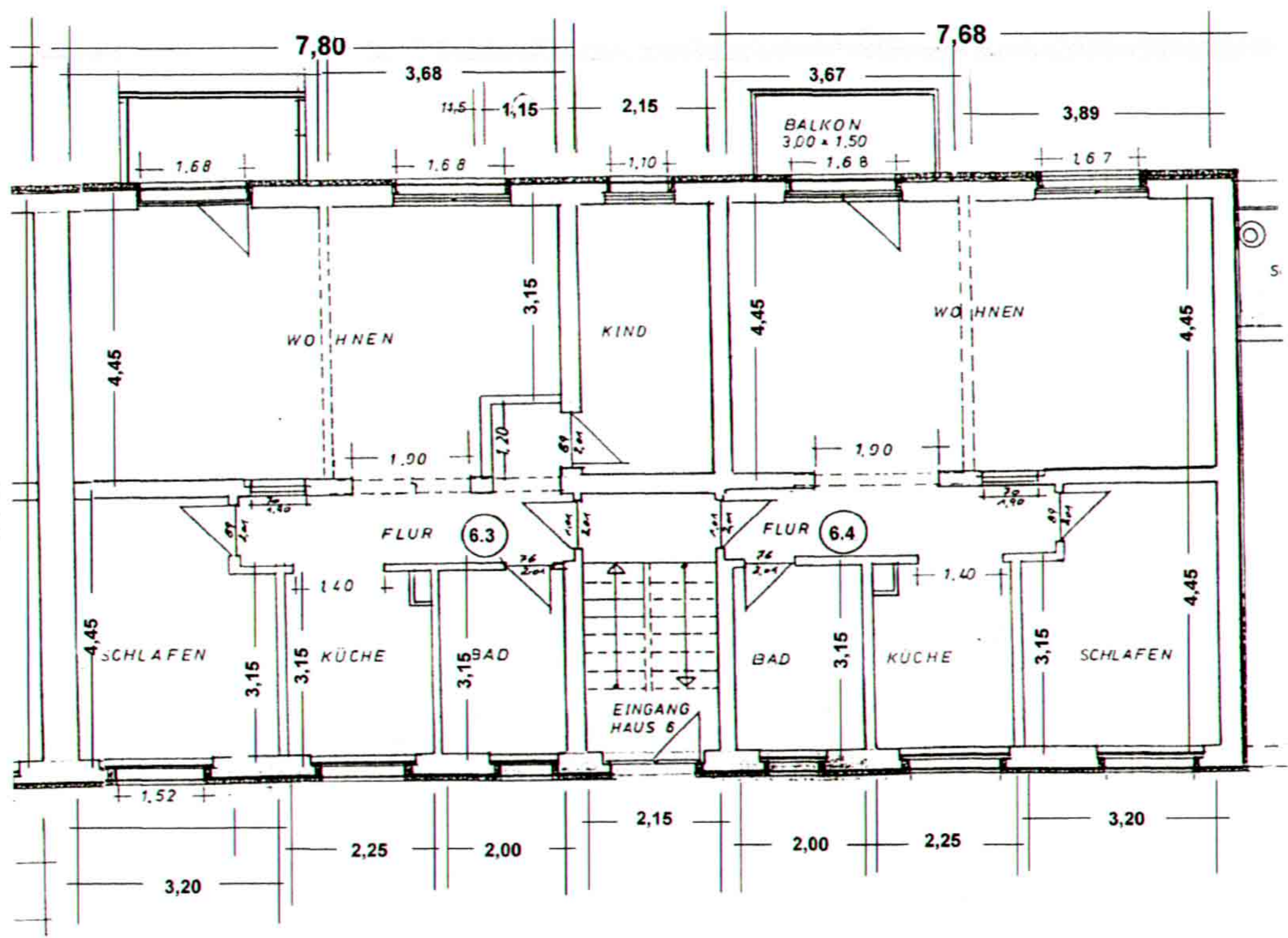
Oybin, Lückendorferstrasse 6 Grundriss Wohnungen 6.3 und 6.4 OBERGESCHOSS
