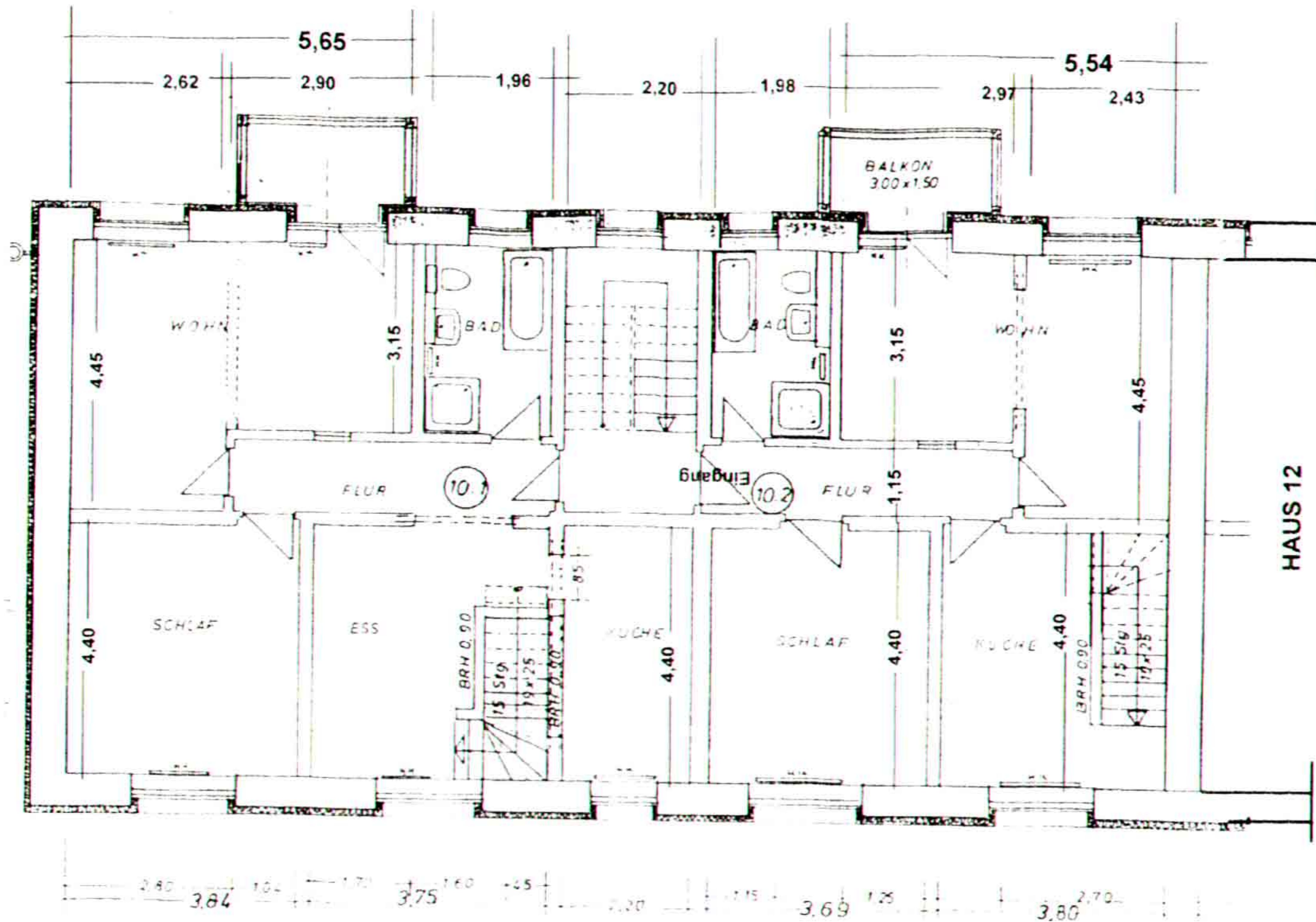
Oybin, Lückendorferstrasse 10 Grundriss Wohnungen 10.1 und 10.2 ERDGESCHOSS
