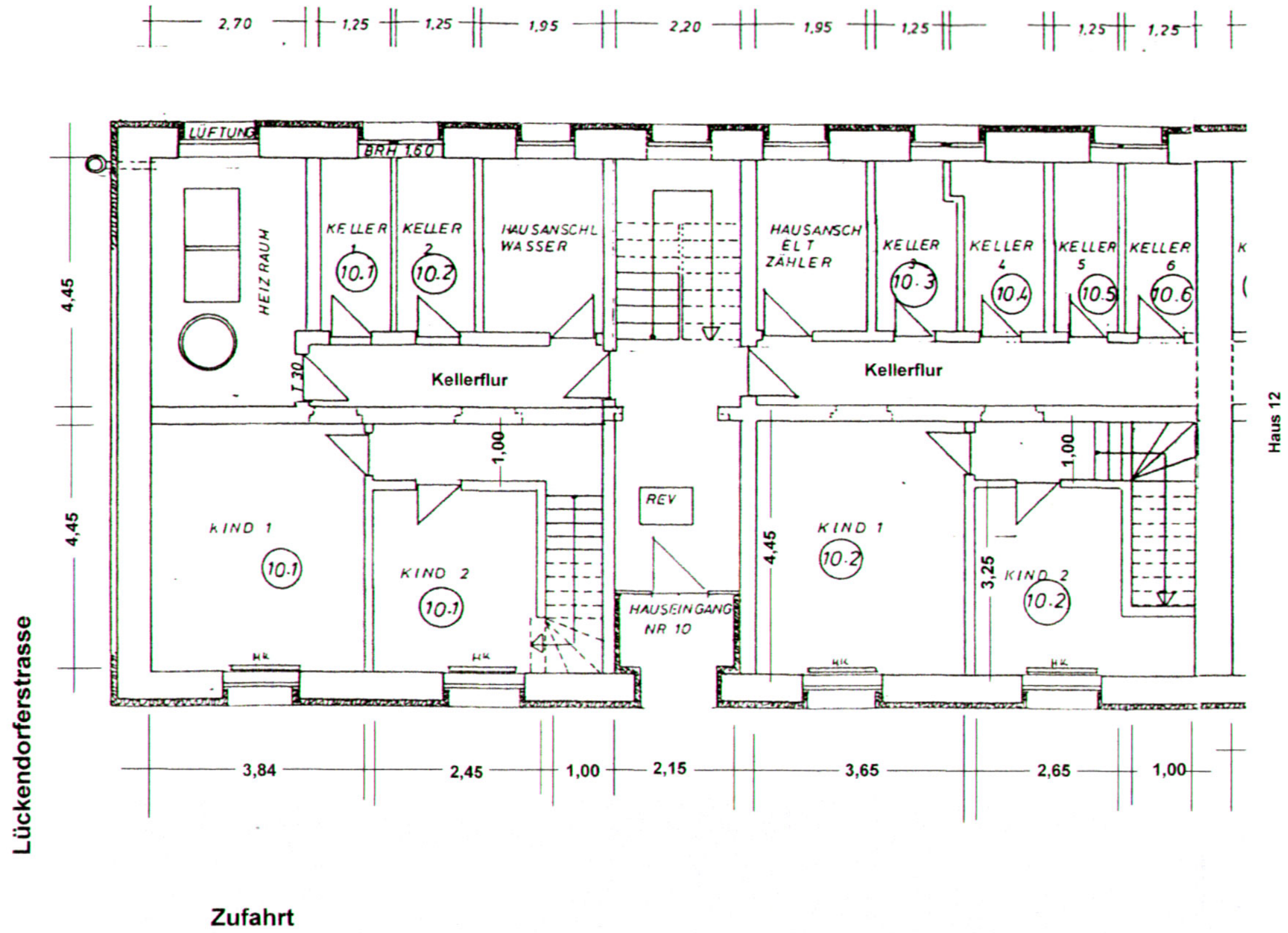
Oybin, Lückendorferstrasse 10 Grundriss Wohnungen 10.1 und 10.2 UNTERGESCHOSS
